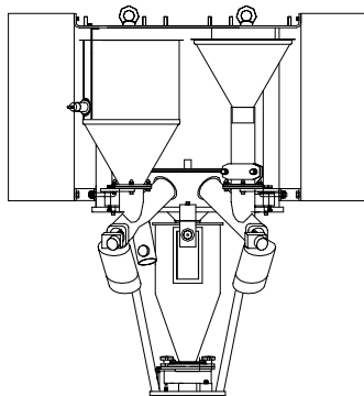
KONTINUIERLICHER MISCHER MIT PCCWEB®
